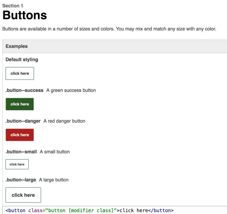
图 10-3 带变体的按钮模块
